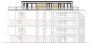
Linker zijgevel
